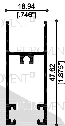
19444 ZOCLO - CABEZAL
