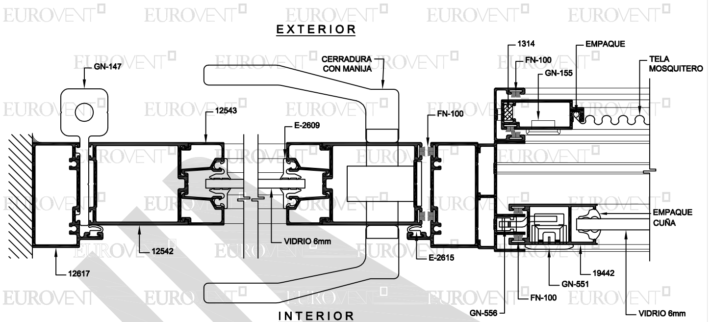
SECCIÓN 21
