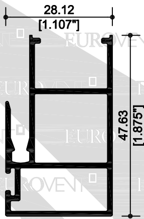
19443 TRASLAPE
