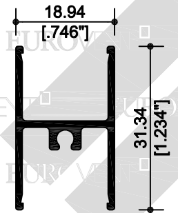
19973 INTERMEDIO
