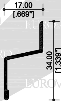
12428 BOTAGUAS
