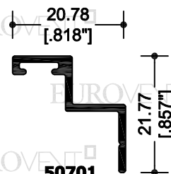
50701 ADAPTADOR OXO
