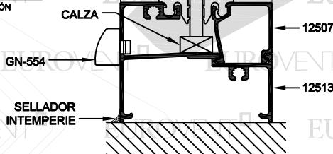
SECCIÓN 15 OPCIÓN
