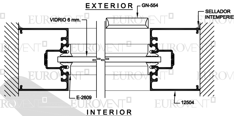
SECCIÓN 12
