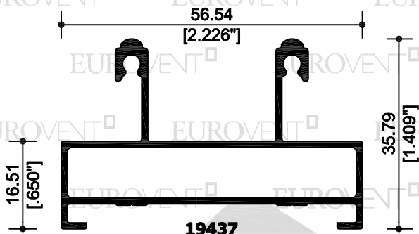
19437 RIEL - CABEZAL
