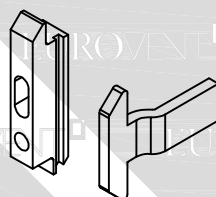
GN-556 CONTRA Y GANCHO
