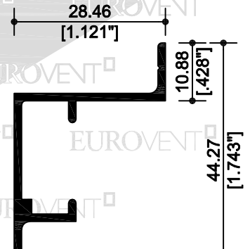
11409 CABEZAL P/MOSQUITERO
