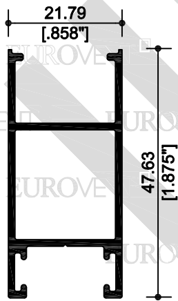
19442 CERCO
