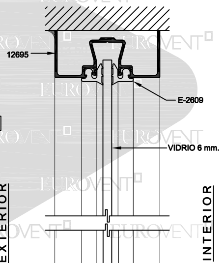
SECCIÓN 16
