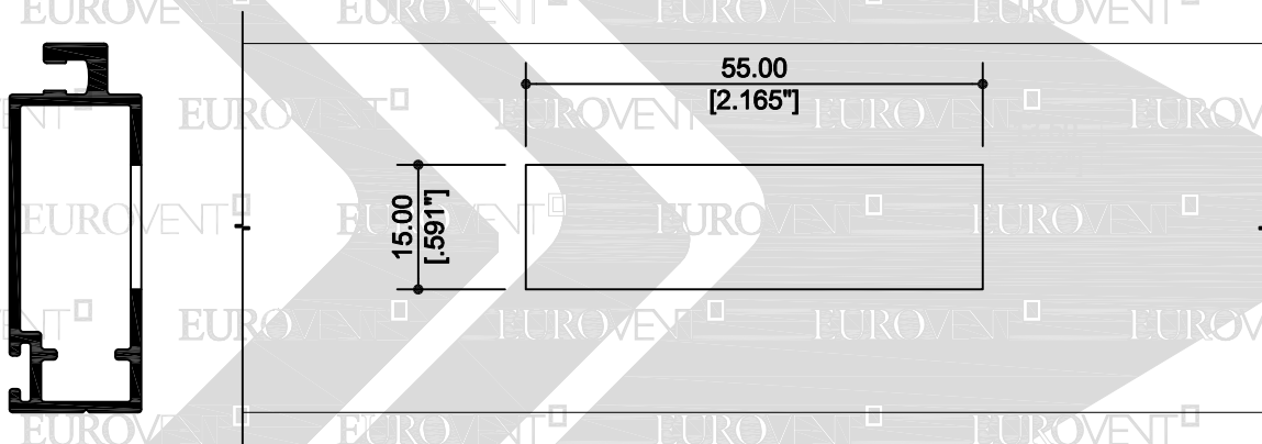
18930 MOSQUITTO UÑERO
