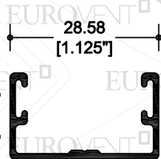
19948 GUÍA INFERIOR
